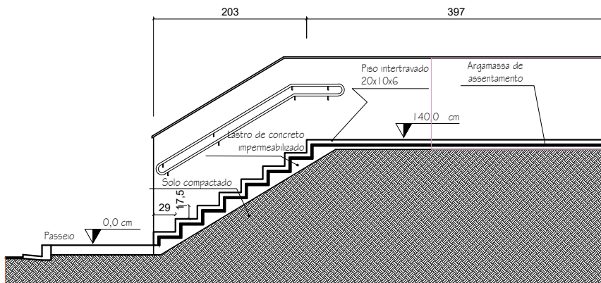
CORTE AA
