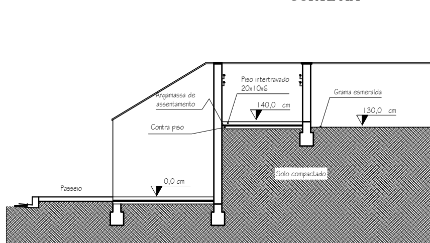
CORTE BB
